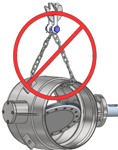
Abbildung 4-4: Anschlag durch das Armaturengehäuse
