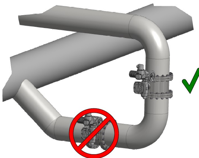
Abbildung 5-2: Position in der Rohrleitung / 2
