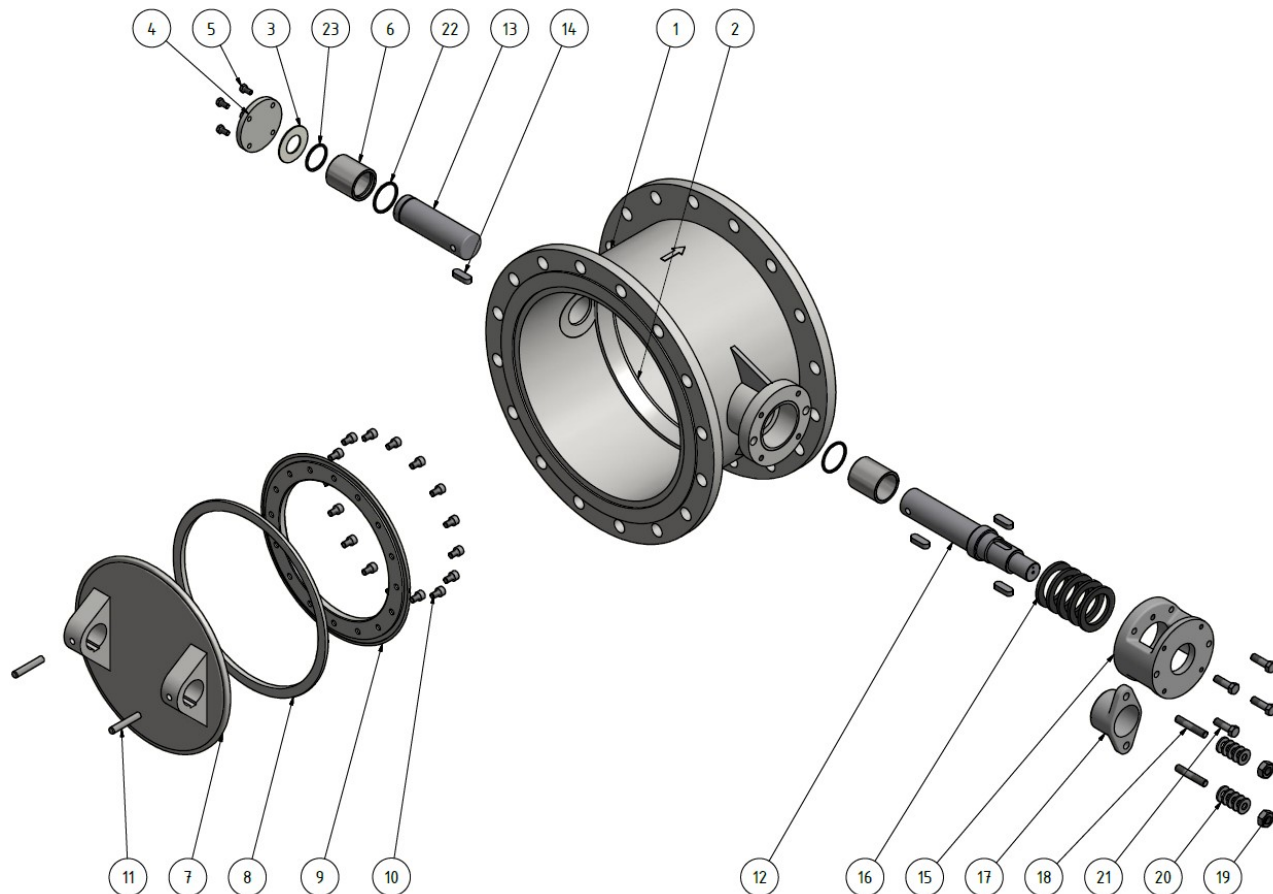
Abbildung 3-1: exemplarische Abbildung einer Absperrklappe
