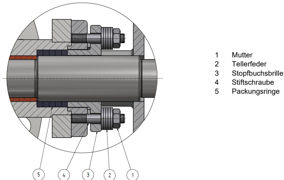
Abbildung 7-2: Stopfbuchse
