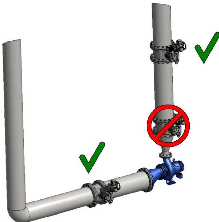
Abbildung 5-1: Position in der Rohrleitung / 1
