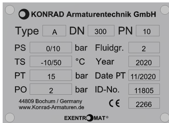
Abbildung 3-3: Typenschild
