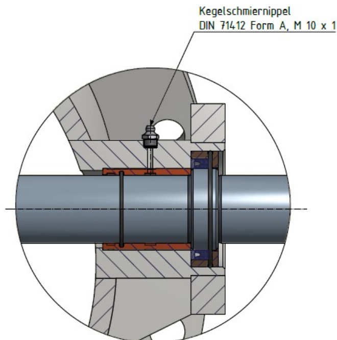
Abbildung 7-1: Fettsperkkammer
