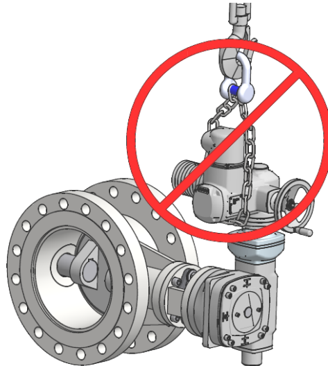
Abbildung 4-3: Anschlag am Antrieb
