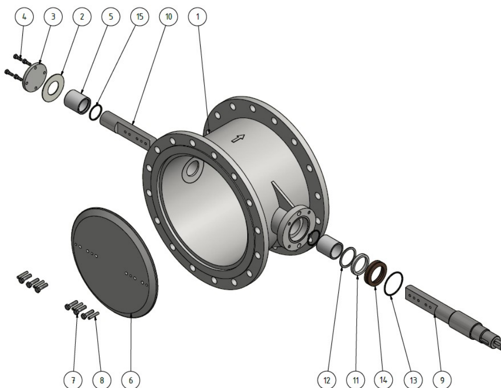
Abbildung 3-2: exemplarische Abbildung einer Drosselklappe
