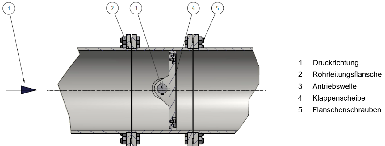
Abbildung 5-3: Querschnitt Absperrklappe
