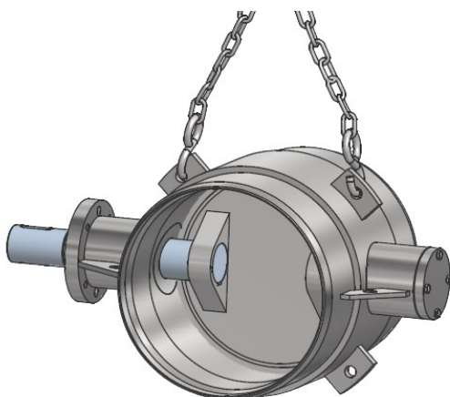
Abbildung 4-1: Anschlag an den Kranösen
